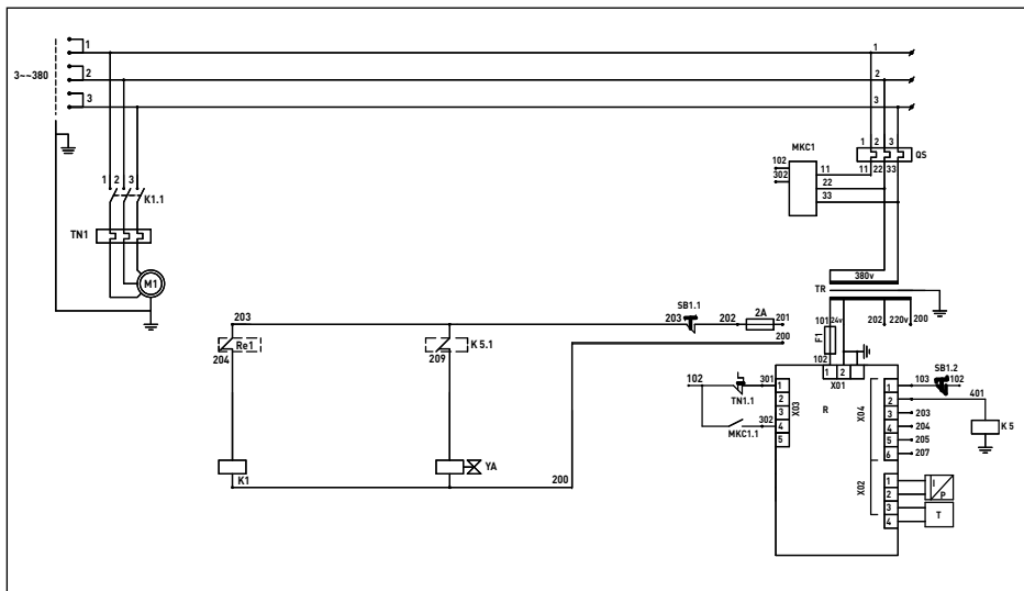
Bild 2.4 Elektro-Schaltplan A07..., AR07..., ARD07...*
