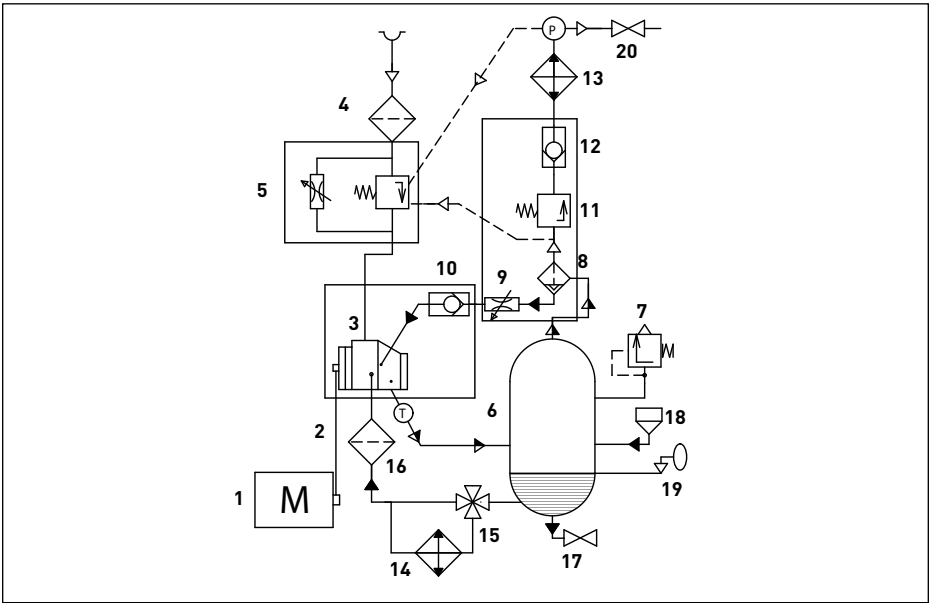
Bild 2.1 Ablaufdiagramm A07..-A22..
