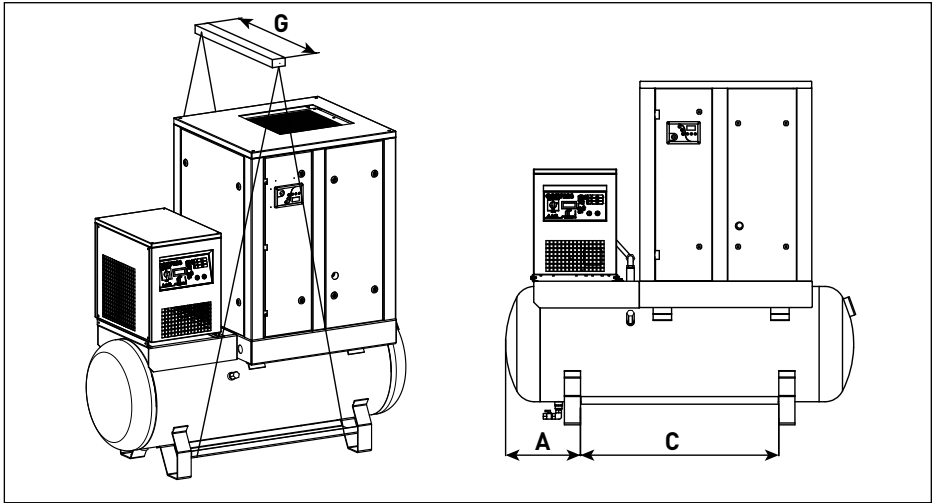
Fig. 3.2 Heben und Transportieren AR07..-AR22, ARD07..-ARD22
