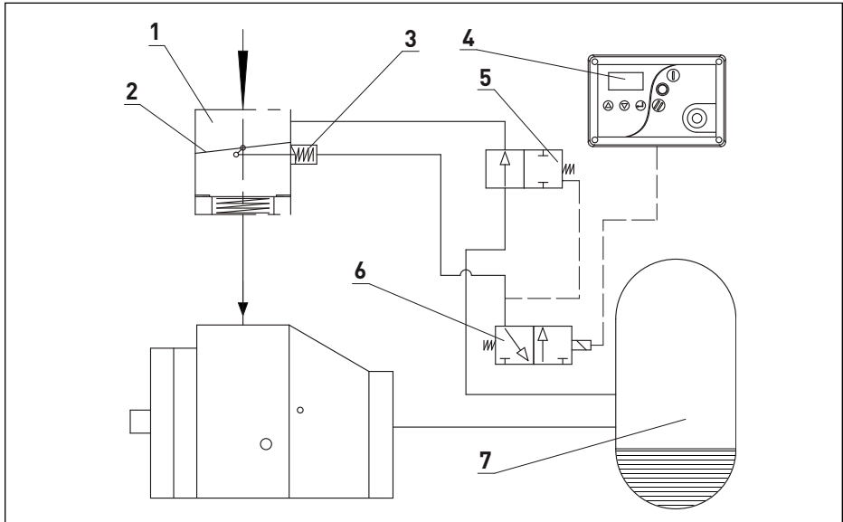
Рис. 2.5 Система регулювання
