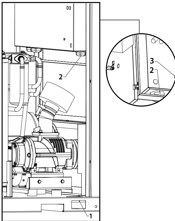
Bild 3.5 Stromkabelverbindung
