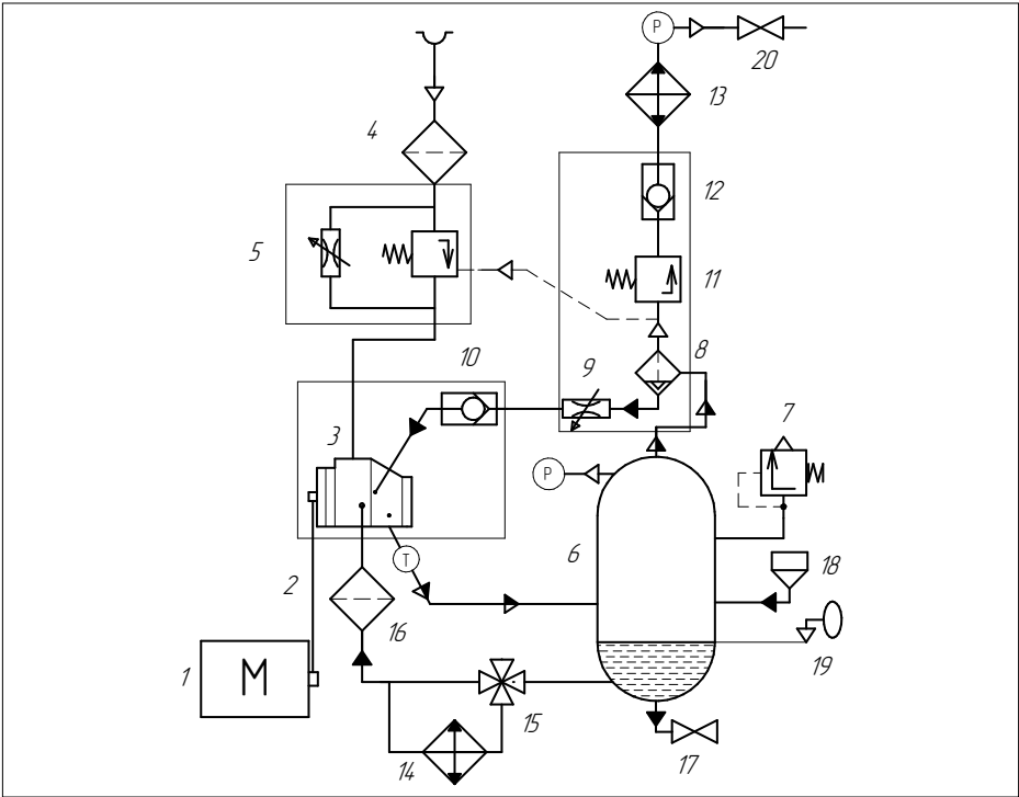
Bild 2.3 Ablaufdiagramm A75-90
