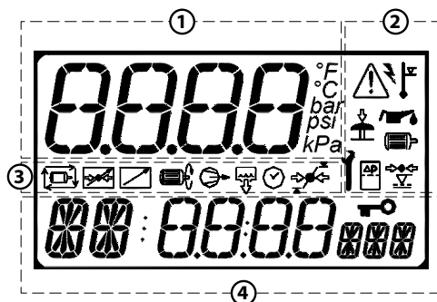
Рис. 4.2 LCD дисплей.
