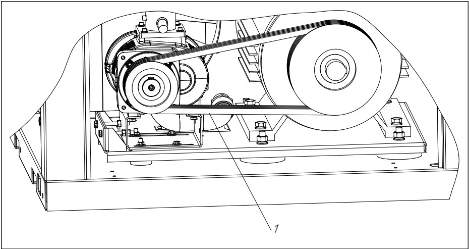
Bild 5.3 Überprüfung des Antriebsriemens
