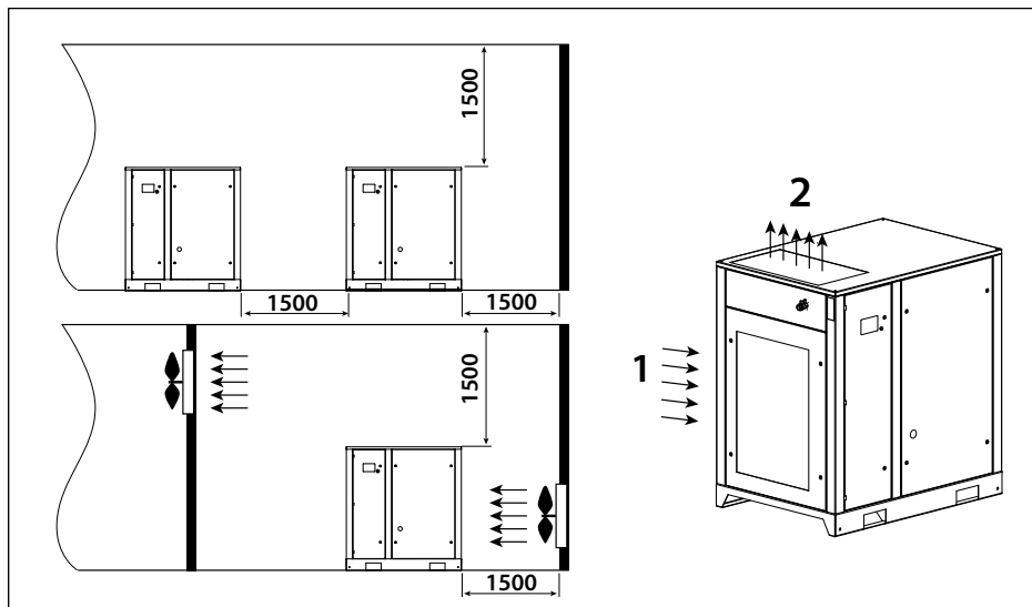
Рис. 3.3 Схема установки компрессора A30 – A55
